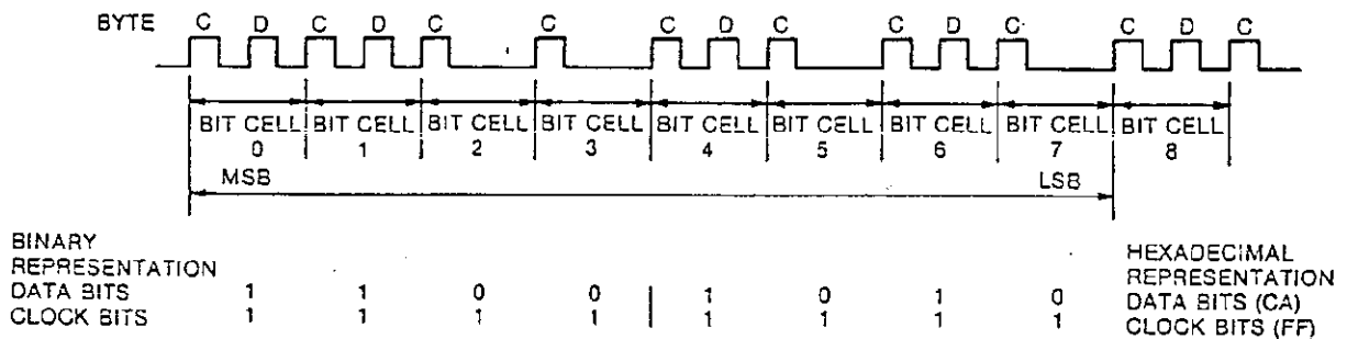
FIGURE 6-1. BYTE (FM ENCODING)
